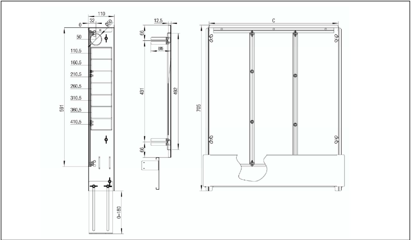
Imag. 9-21 Dimensiuni dulap de distribuție UP C Lățime carcasă interioară
